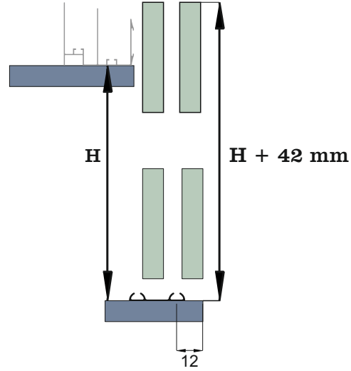
YAN GÖRÜNÜM / SIDE VIEW
