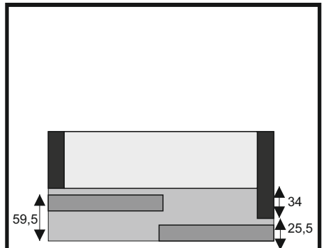
ÖN GÖRÜNÜM / FRONT VIEW
