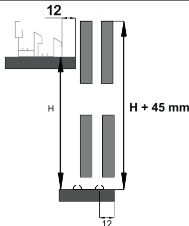
YAN GÖRÜNÜM / SIDE VIEW
